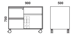
Combo Unit -FF/Open
